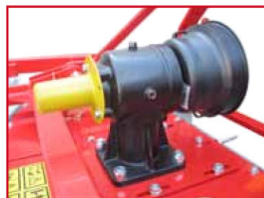
Renvoi d'angle à double sens de rotation
